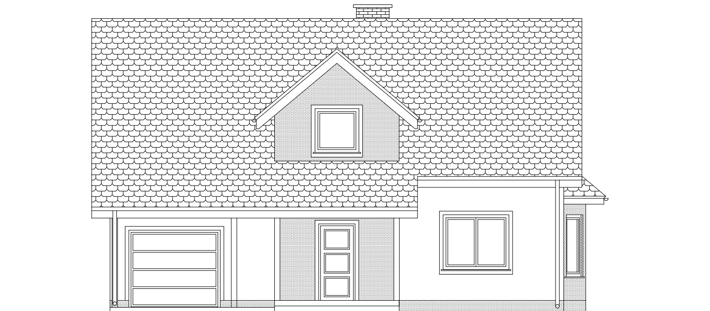
ELEWACJA FRONTOWA
