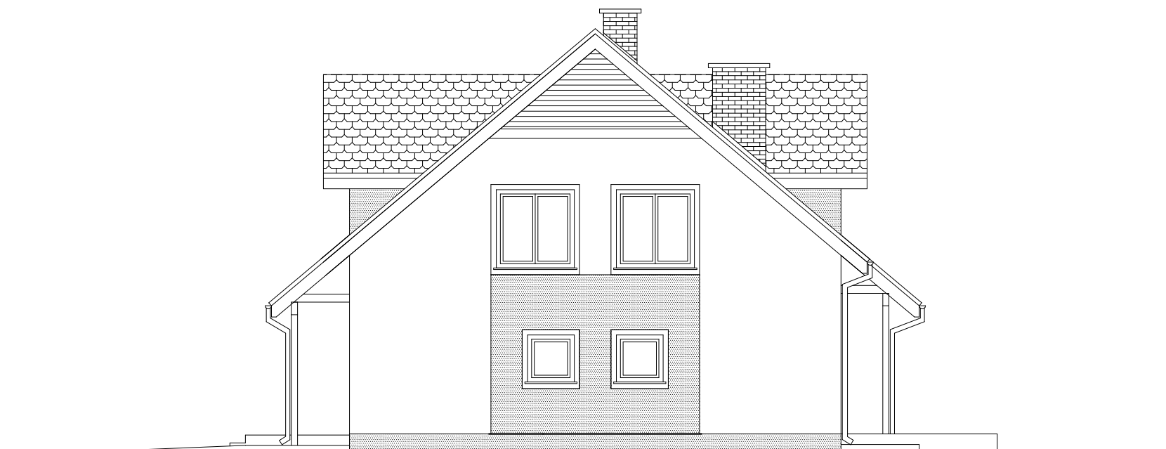
ELEWACJA BOCZNA
