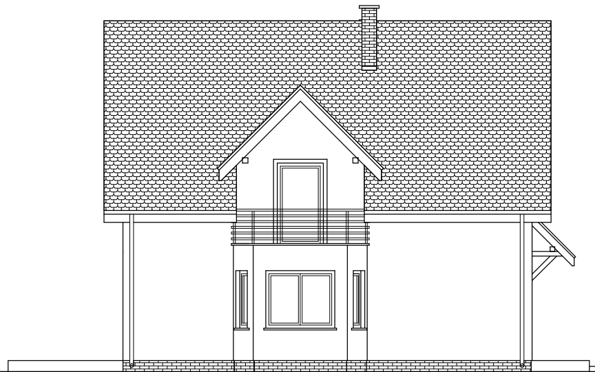
ELEWACJA BOCZNA
