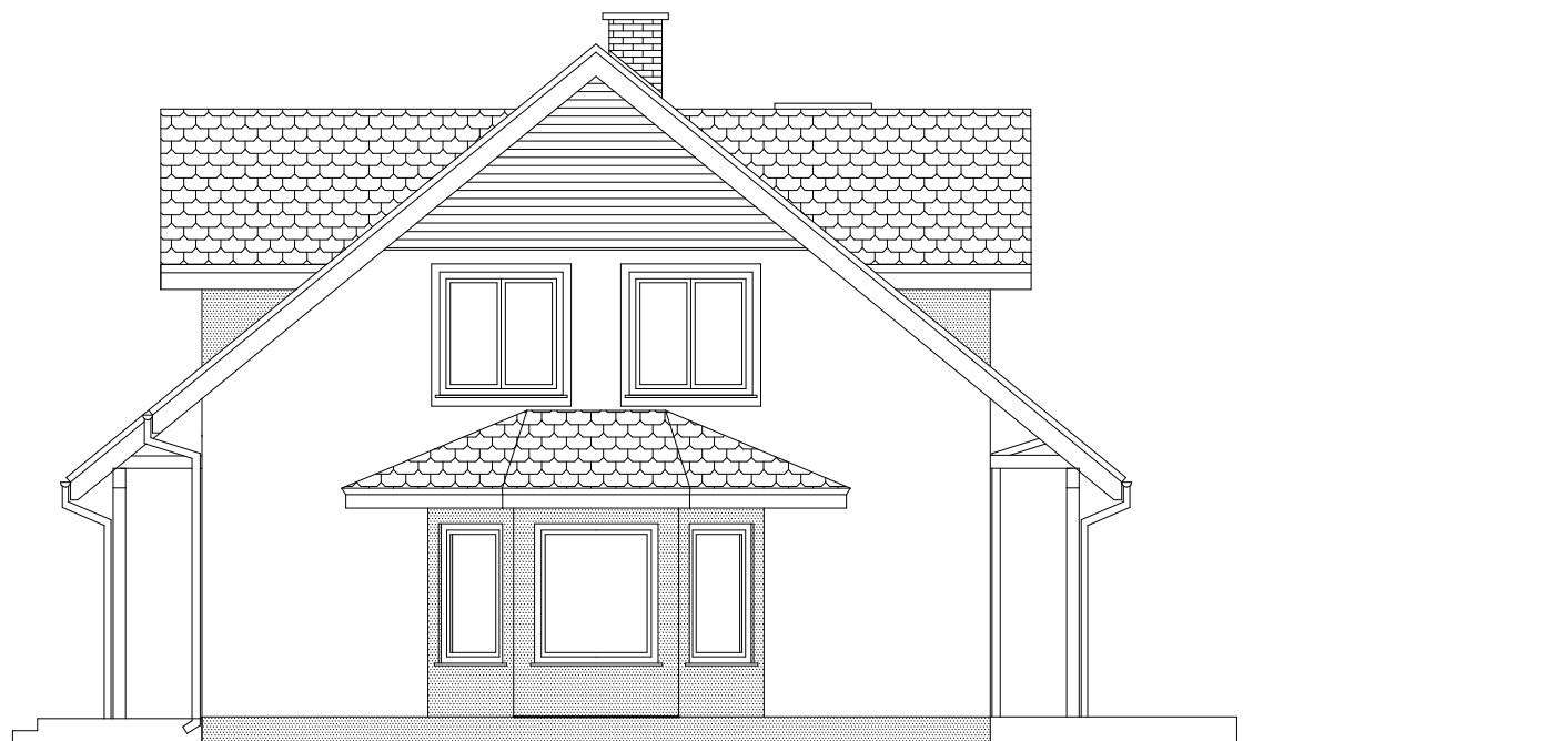
ELEWACJA BOCZNA
