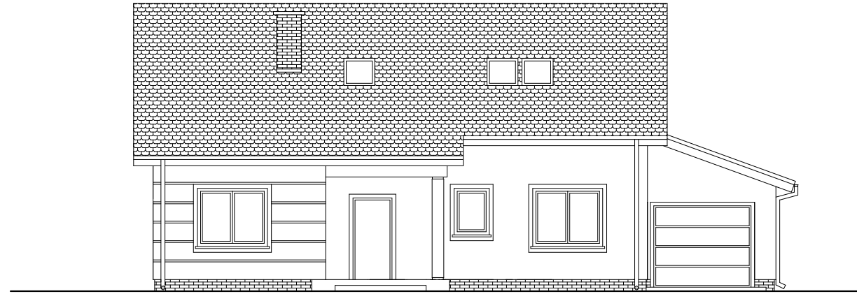
ELEWACJA FRONTOWA
