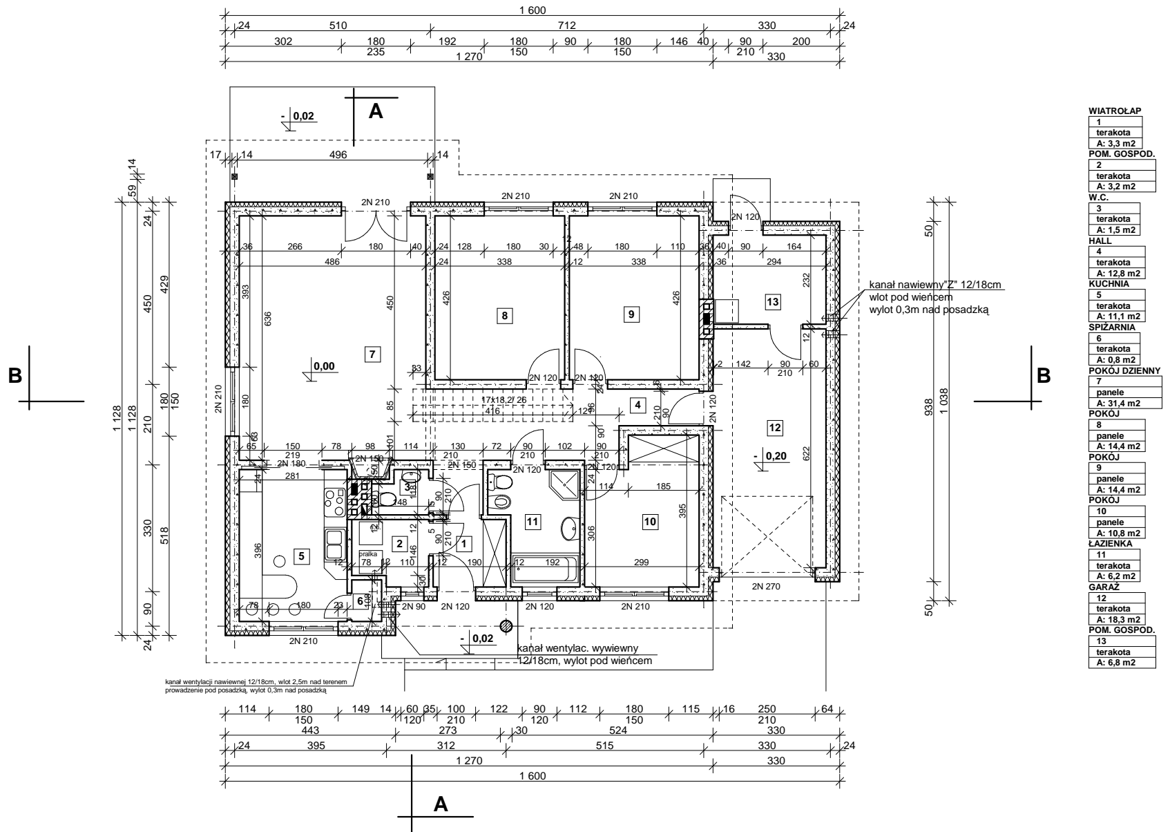
PARTER "A" POWIERZCHNIA UŻYTKOWA PARTERU = 110,2 m 2 + garaż i pom. gospod. = 25,1 m 2
