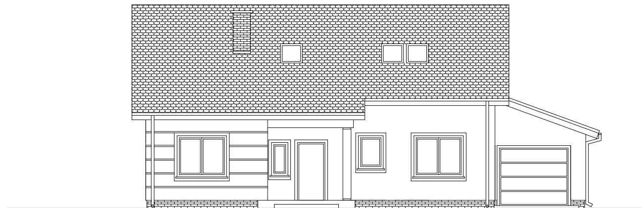
ELEWACJA FRONTOWA
