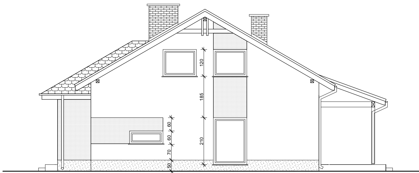
ELEWACJA BOCZNA
