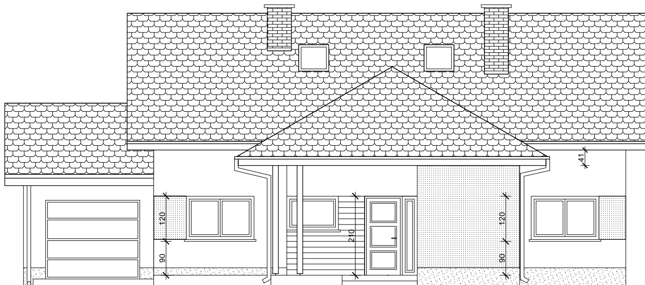
ELEWACJA FRONTOWA
